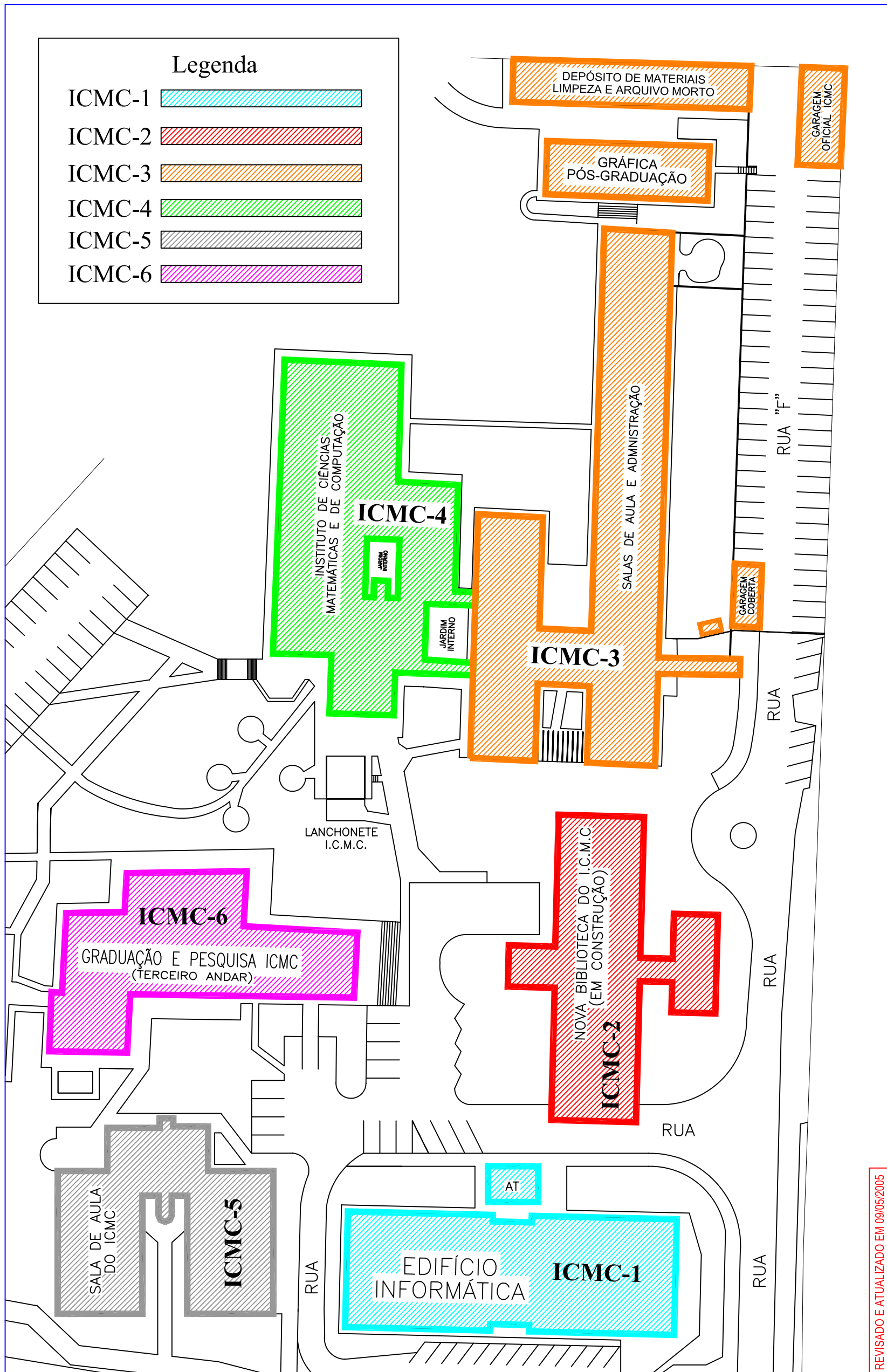
PREFEITURA DO CAMPUS ADMINISTRATIVO DE SÃO CARLOS - USP PLANTA DE LOCALIZAÇÃO DOS PRÉDIOS DO I.C.M.C.
